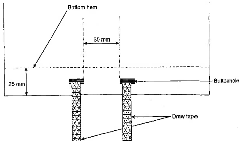
Fig 9 - Bottom
